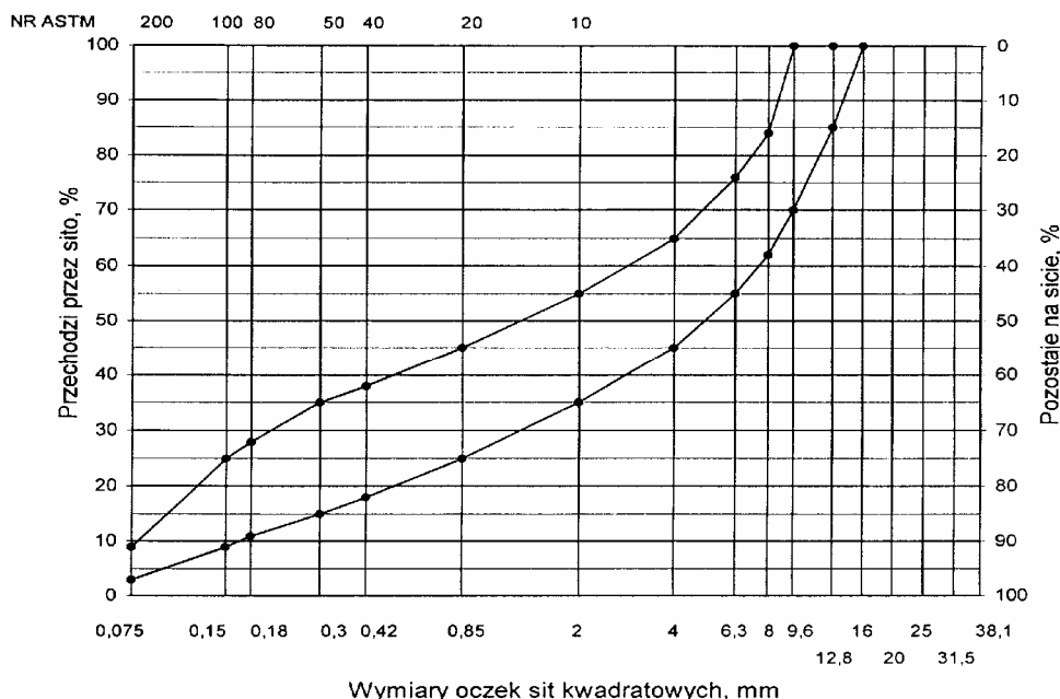
Rys. 7. Krzywe graniczne uziarnienia mieszanki mineralnej BA od 0 do 12,8 mm do warstwy wiążącej, wyrównawczej i wzmacniającej nawierzchni drogi o obciążeniu ruchem KR1 lub KR2 Tablica 6. Wymagania wobec mieszanek mineralno-asfaltowych i warstwy wiążącej, wyrównawczej oraz wzmacniającej z betonu asfaltowego
