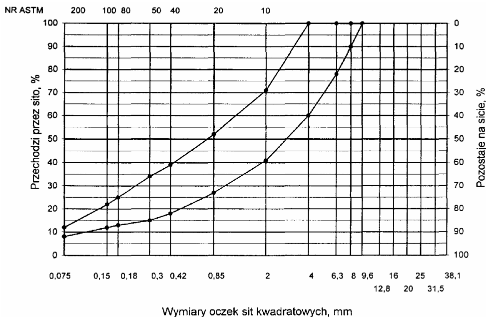
Rys. 2. Krzywe graniczne uziarnienia mieszanki mineralnej BA od 0 do 16mm, od 0 do 12,8 mm
