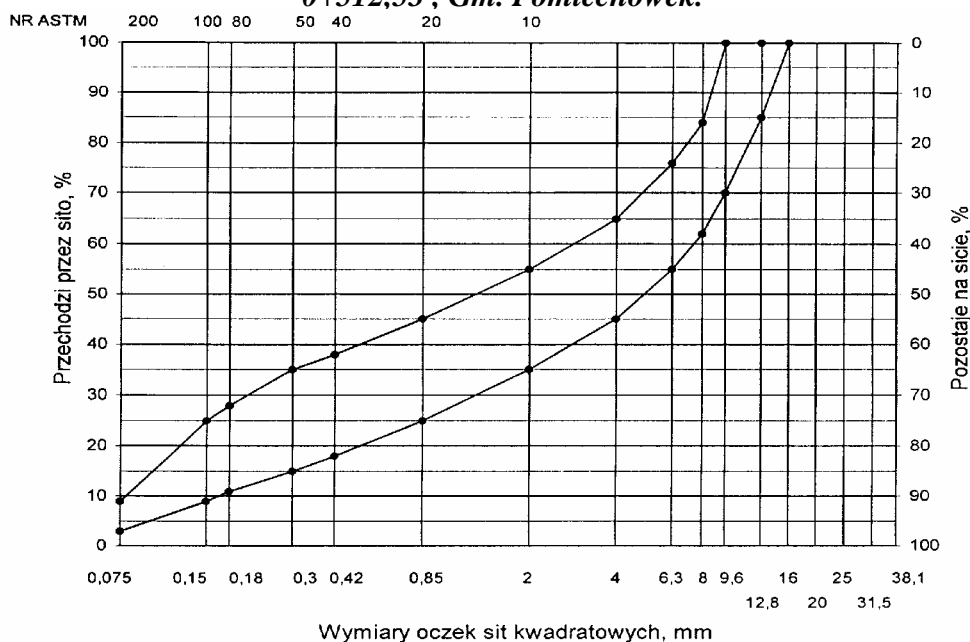
Rys. 7. Krzywe graniczne uziarnienia mieszanki mineralnej BA od 0 do 12,8 mm do warstwy wiążącej, wyrównawczej i wzmacniającej nawierzchni drogi o obciążeniu ruchem KR1 lub KR2
