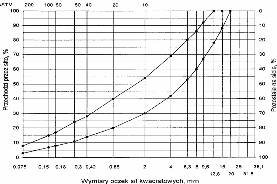
Rys. 5. Krzywe graniczne uziarnienia mieszanki mineralnej BA od 0 do 20 mm do warstwy wiążącej, wyrównawczej i wzmacniającej nawierzchni drogi o obciążeniu ruchem KR1 lub KR2
