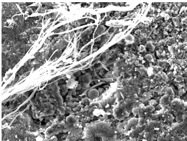
Rys. 4. Korozja płyt a-c – widoczna wiązka całkowicie odstłoniętych włókien (pow. 400x) (wg J.Dyczek)
